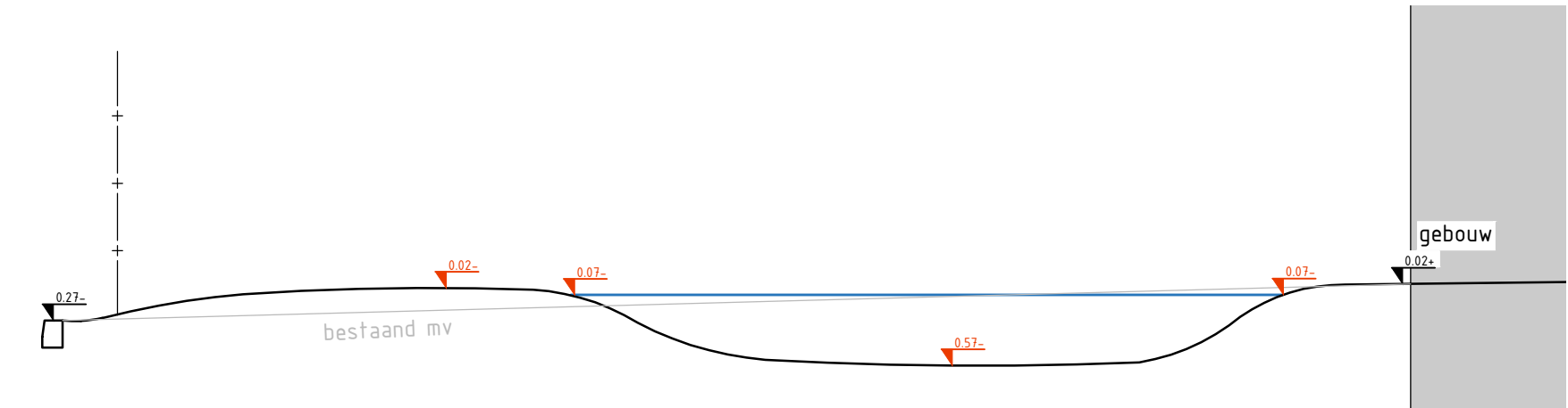
Principe doorsnede 1 schaal 1:50
