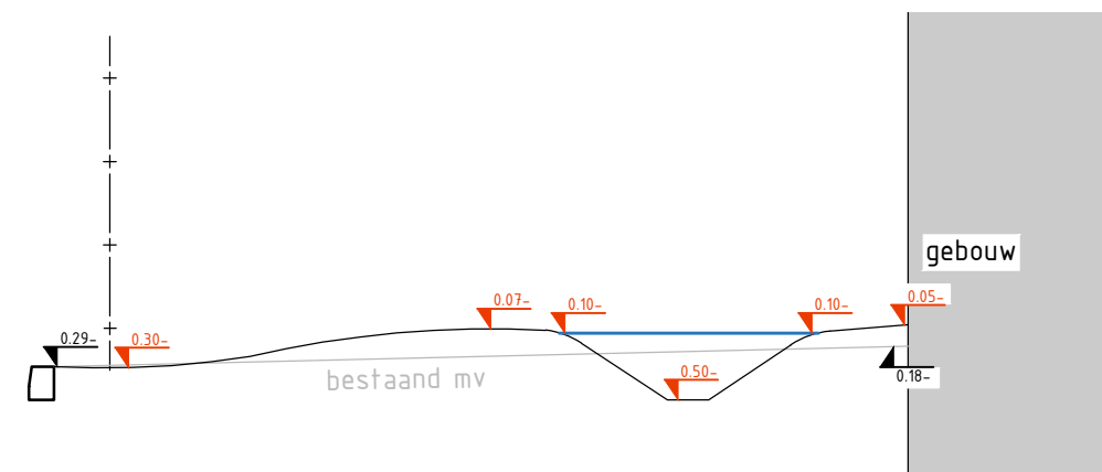
Principe doorsnede 5 schaal 1:50
