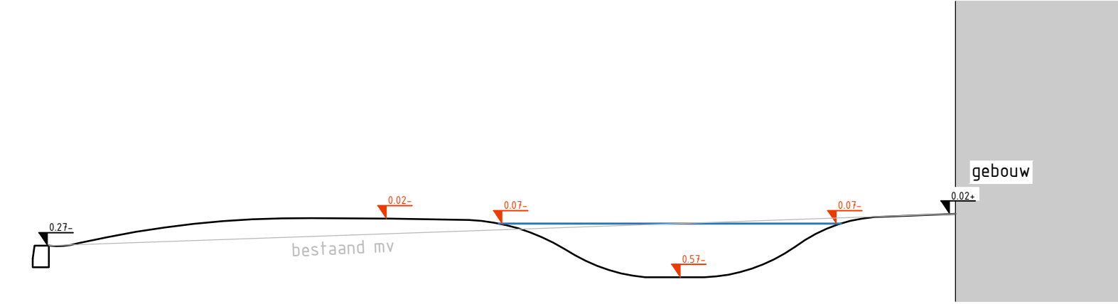
Principe doorsnede 2 schaal 1:50
