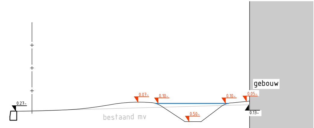
Principe doorsnede 3 schaal 1:50
