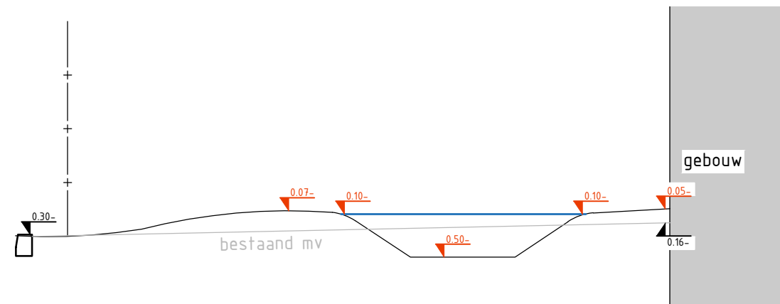
Principe doorsnede 4 schaal 1:50
